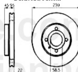
5. BS 100615 hinten/rear
