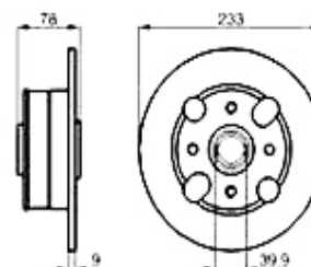
5. BS 100615 hinten/rear
