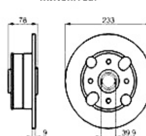
5. BS 100615 hinten/rear
